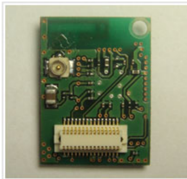
AZEL-N01コネクタ面
